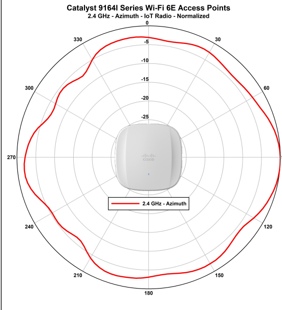
Figure 15: CW9164I - IoT (BLE) アンテナ正規化放射パターン (2.4 GHz 水平)
