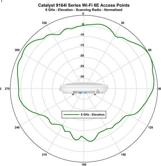
Figure 14: CW9164I - スキャン無線正規化放射パターン (6 GHz 垂直)
