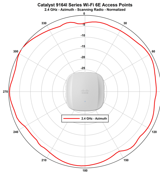
Figure 9: CW9164I - スキャン無線正規化放射パターン (2.4 GHz 水平)
