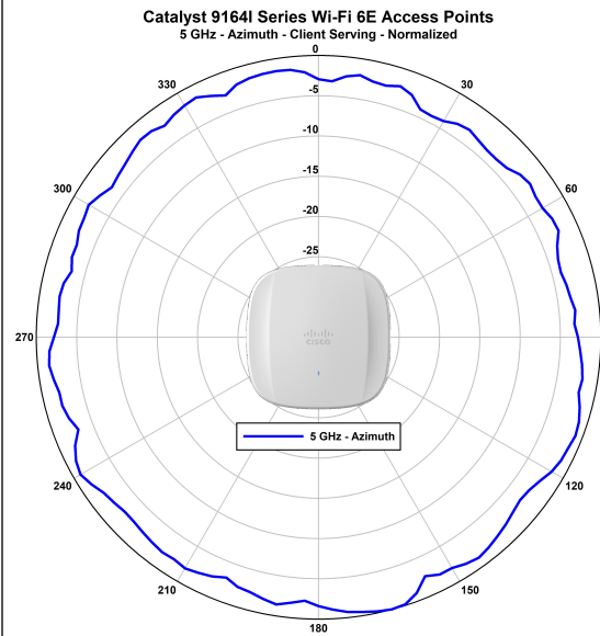
Figure 5: CW9164I - クライアントサービス正規化放射パターン (5 GHz 水平)
