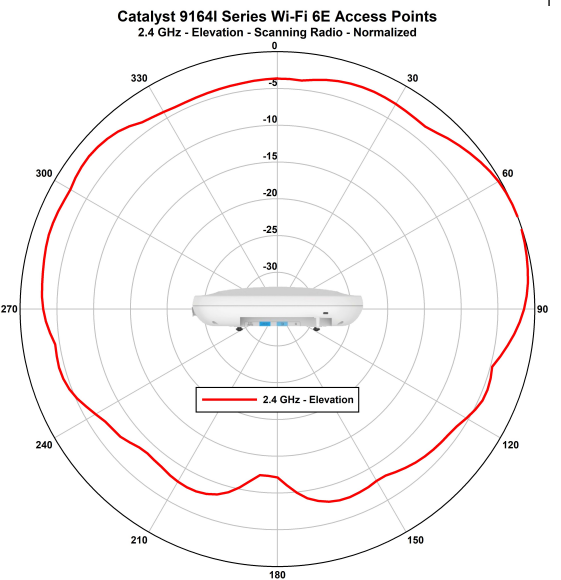
Figure 10: CW9164I - スキャン無線正規化放射パターン (2.4 GHz 垂直)
