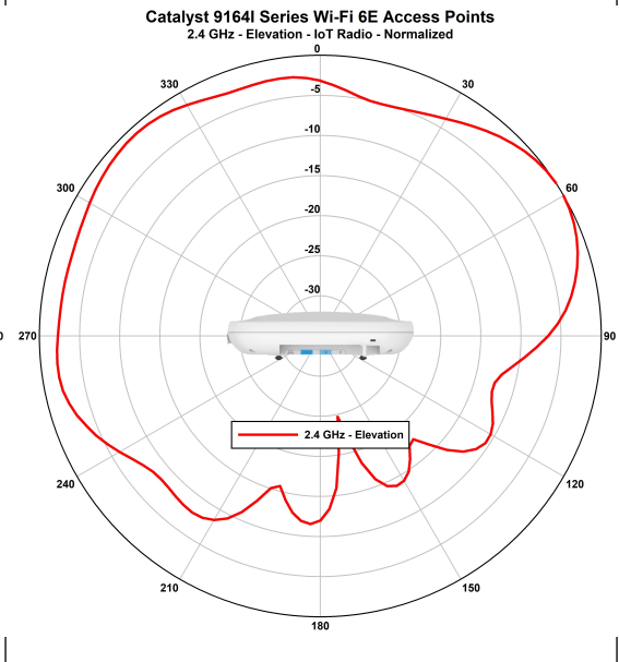
Figure 16: CW9164I - IoT (BLE) アンテナ正規化放射パターン (2.4 GHz 垂直)
