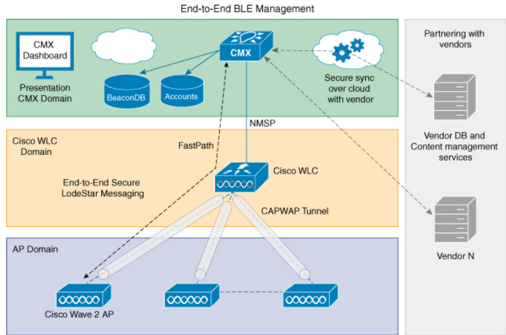
図 26: エンドツー エンドの BLE の管理
