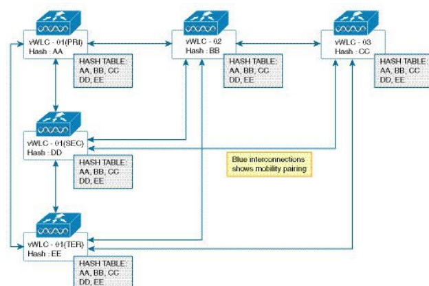
図 17: モビリティ グループ内の vWLC N+1
