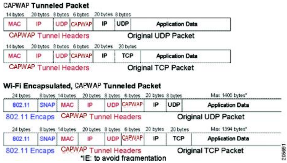
図 60: CAPWAP でトンネリングされたパケット
