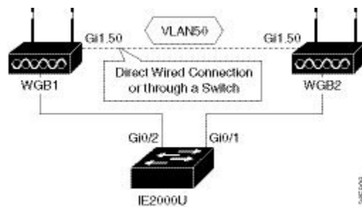
図 74: 2つの WGB 間のピアリンク
