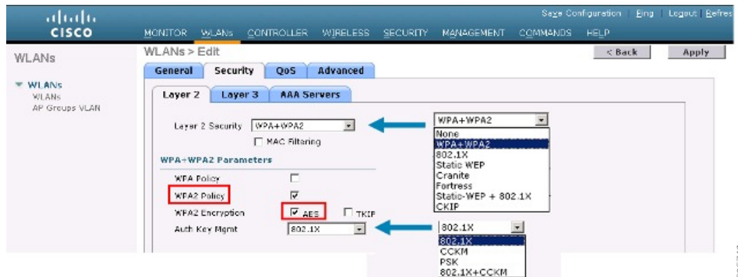
図 33: WGB の WPA-2 セキュリティ設定
