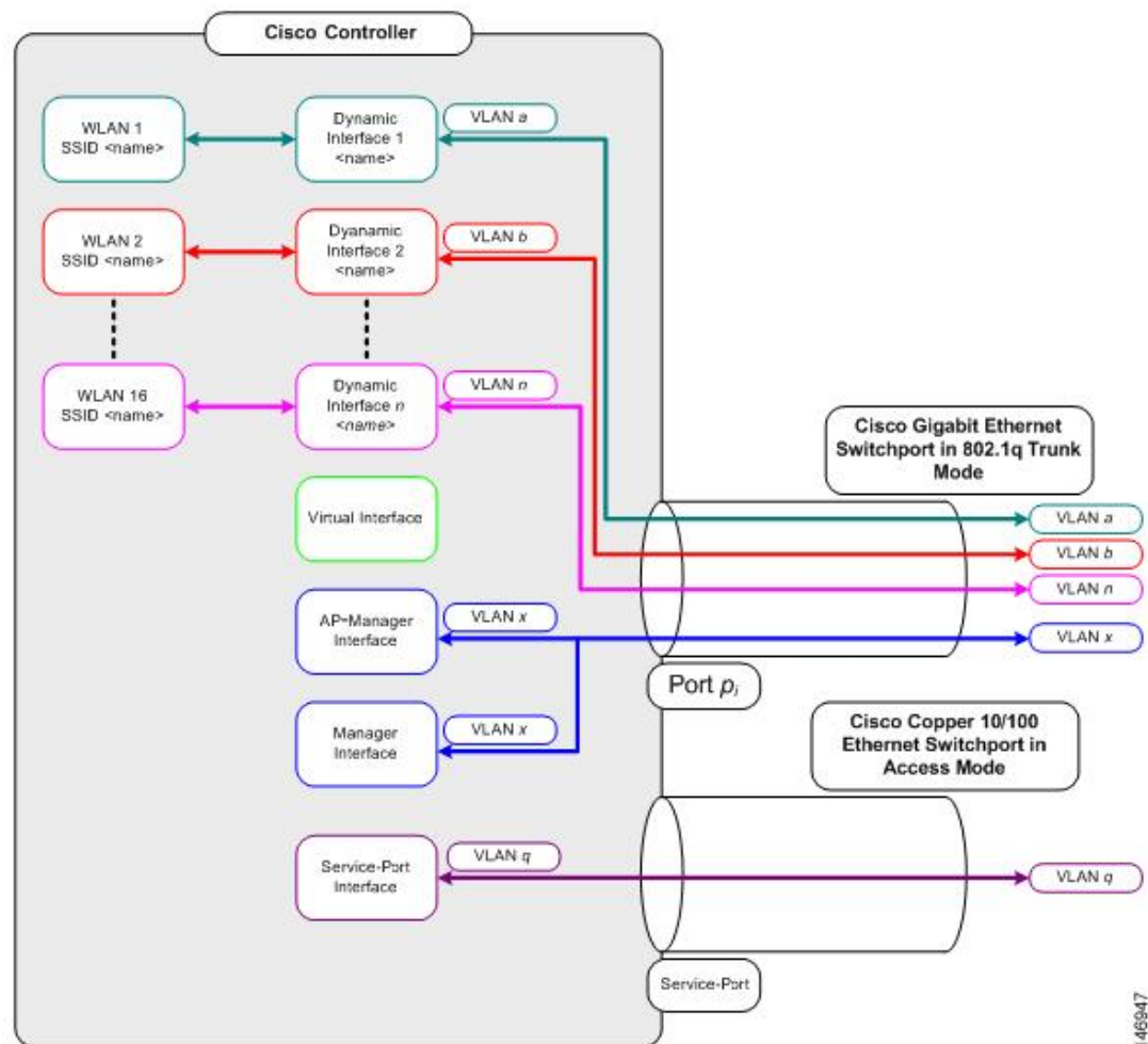
図 19: ポート、インターフェイス、および WLAN の関係
