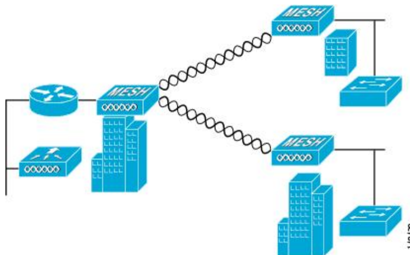
図 29: ポイントツーマルチポイントブリッジング
