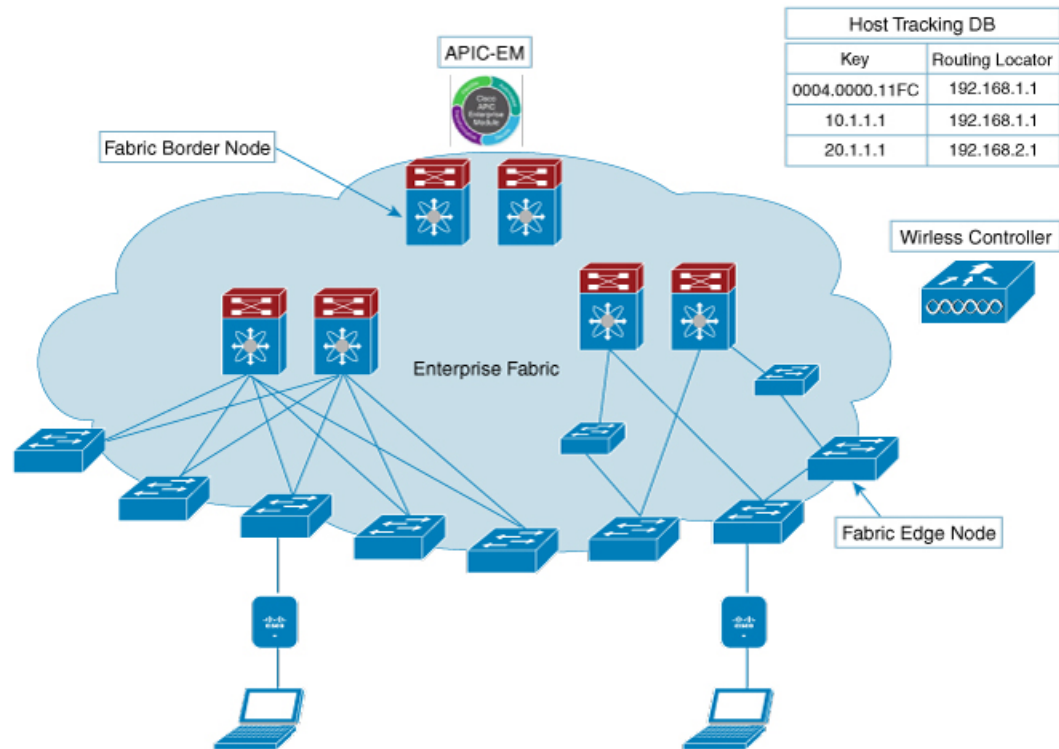
図 76: SD-Access ワイヤレス
