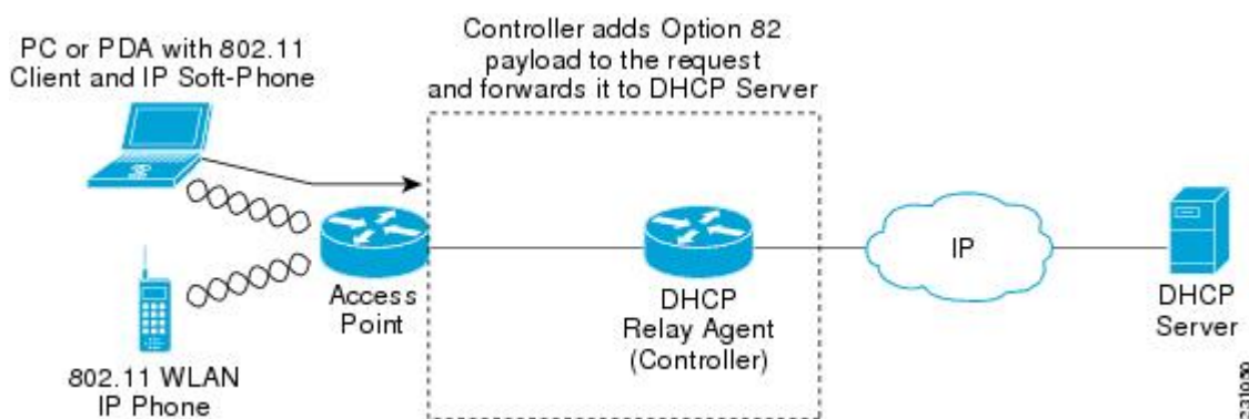
図 67: DHCP オプション 82
