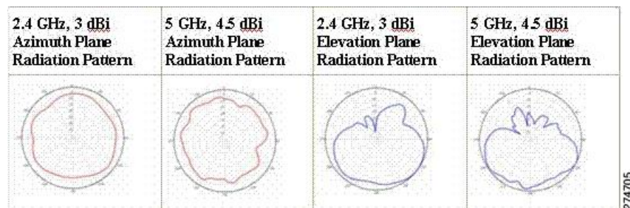
図 87: OfficeExtend アクセスポイントの放射パターン
