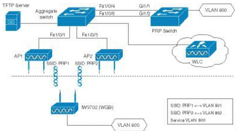
図 75: 1つの PRP スイッチとペアリングされている、デュアル無線がある 1つの WGB 経由での同時ワイヤレス伝送
