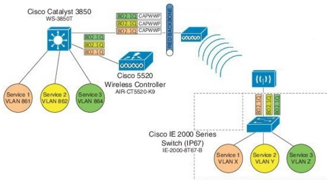
図 72: 複数の VLAN 上のワークグループ ダウンストリーム ブロードキャスト
