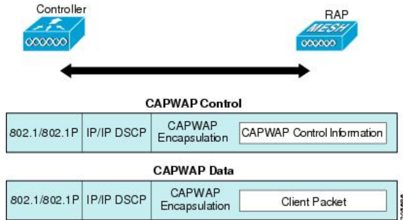
図 27: メッシュ ネットワーク トラフィックの終端
