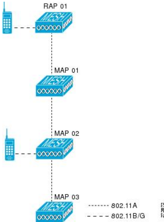
図 46:メッシュ ネットワークの例
