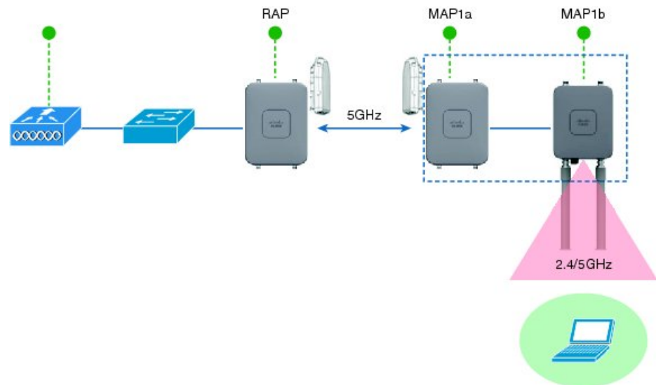
図 52: ユニバーサル アクセスを拡張するデジチェーン接続
