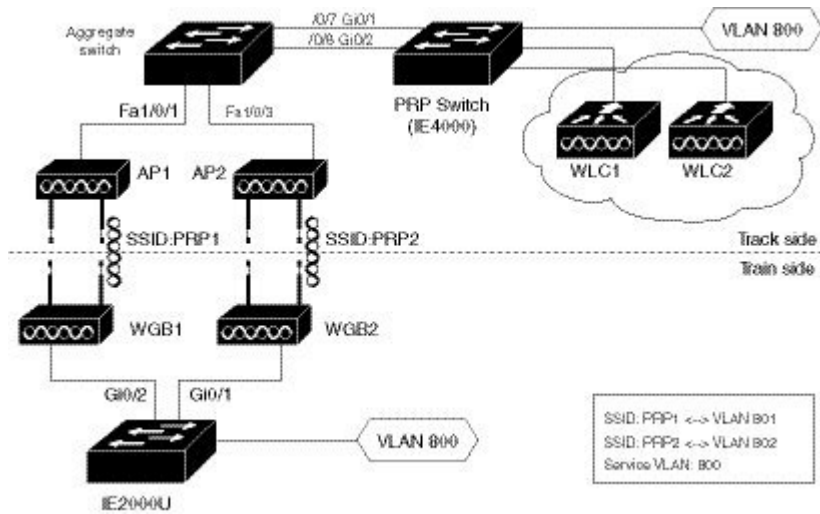
図 73: 1つの PRP スイッチとペアリングされている 2つの WGB 経由での同時ワイヤレス伝送
