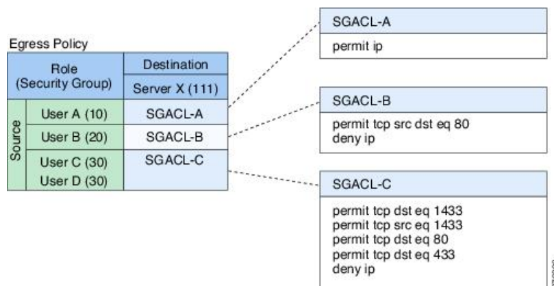
図 20: SGACL ポリシー マトリックスの例
