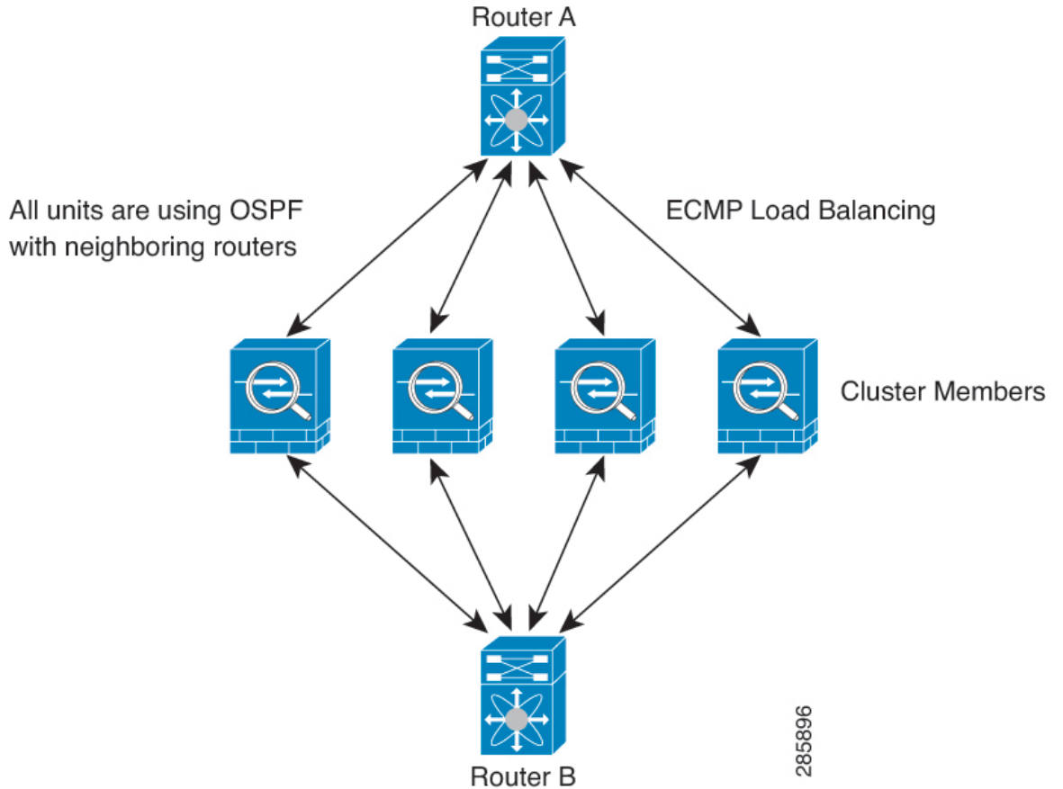
그림 32: 개별 인터페이스 모드의 동적 라우팅
