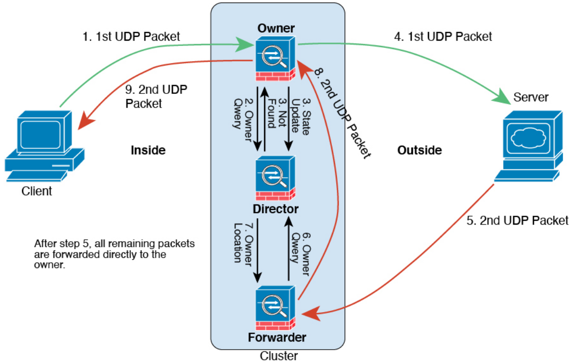
1. 그림 17: ICMP 및 UDP 데이터 플로우
