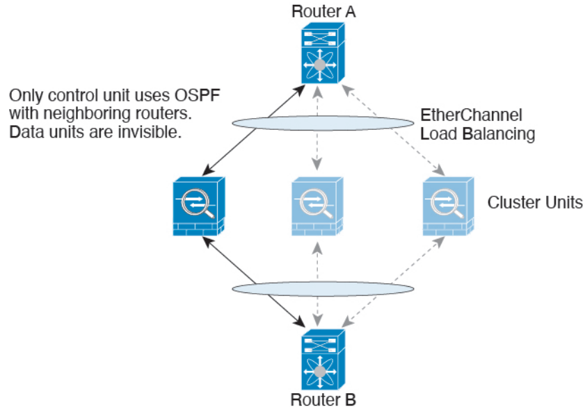
그림 16: 동적 라우팅
