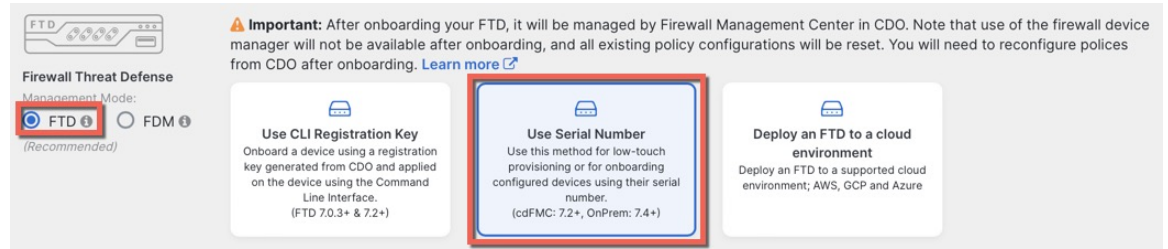
그림 13: 일련 번호 사용
