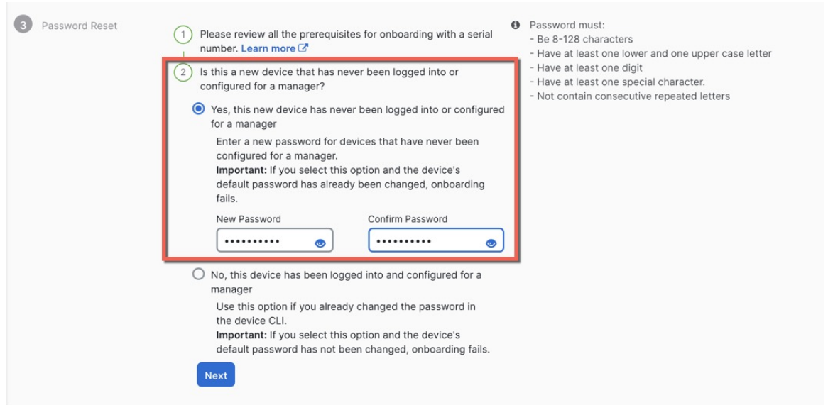
그림 18: Password Reset (비밀번호 재설정)
