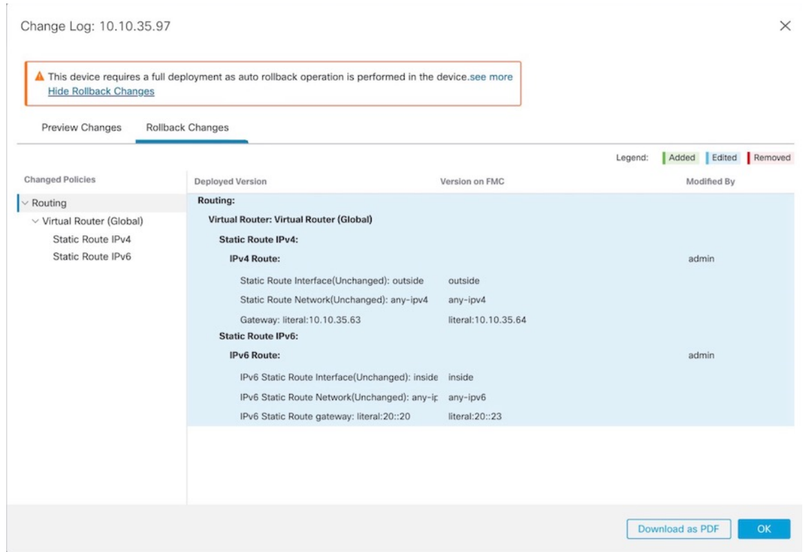
그림 64: 롤백 변경 사항
