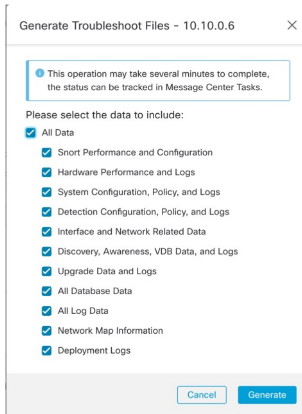
그림 27: 트러블슈팅 파일 생성
