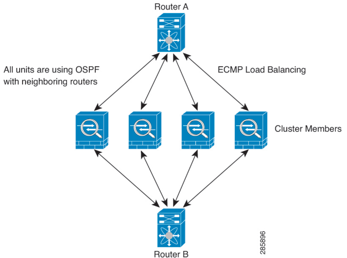
그림 2 개별 인터페이스 모드의 동적 라우팅
