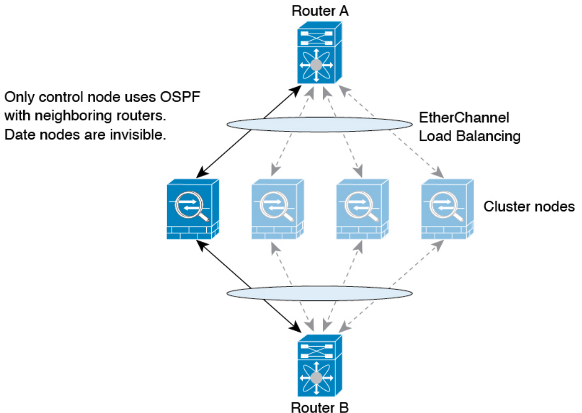
그림 1: Spanned EtherChannel 모드의 동적 라우팅
