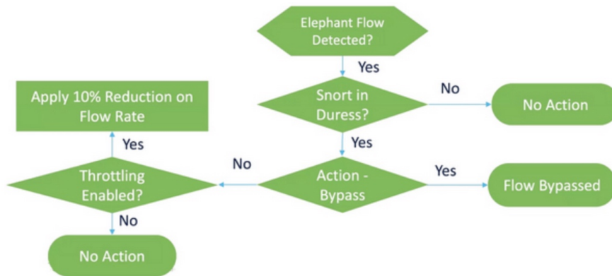
그림 2: 엘리펀트 플로우 워크플로우
