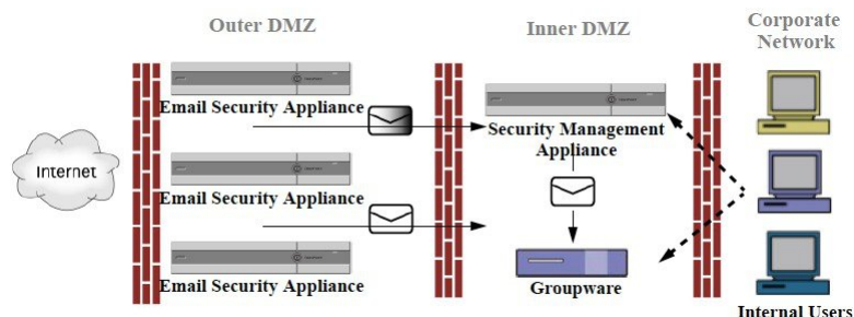
Figure 90: 利用思科安全邮件和 Web 管理器的典型网络配置
