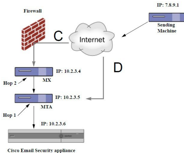
Figure 28: MX/MTA 中继的邮件 - 可变跳数
