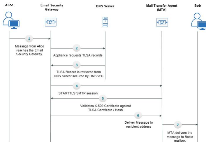
图 46: 使用具有 DANE 支持的 TLS 进行邮件传输
