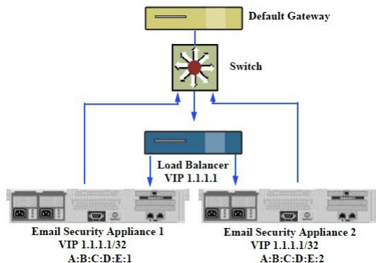
Figure 79: 使用 DSR 实现交换机上多个邮件网关之间的负载均衡
