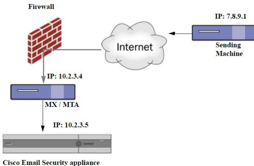
Figure 26: 通过 MX/MTA 中继的邮件 - 简单
