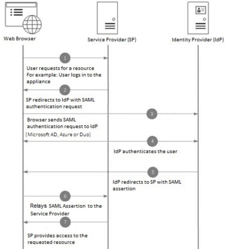
图 3: SAML 工作流
