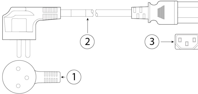
图 23: 以色列 CAB-250V-10A-IS
