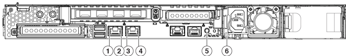
图 13: S195 和 S395 后面板 LED 及其状态
