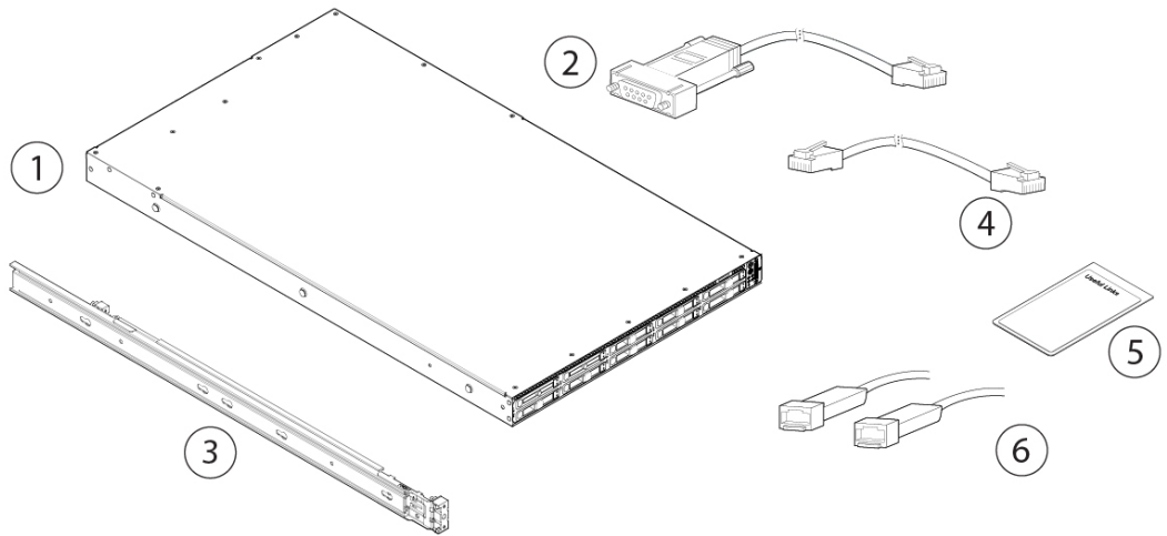
图 3: 装箱清单
