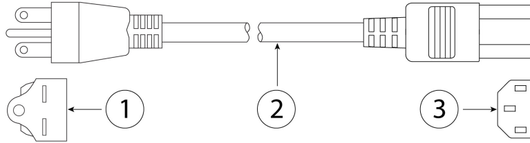
图 29: 北美 CAB-N5K6A-NA
