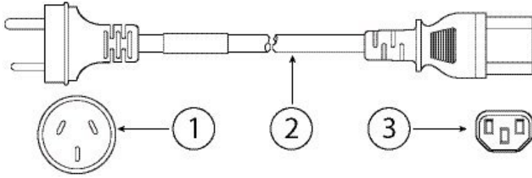
图 20: 中国 CAB-250V-10A-CH
