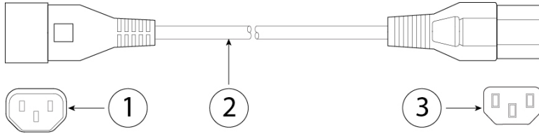
图 26: 日本 CAB-C13-C14-2M-JP
