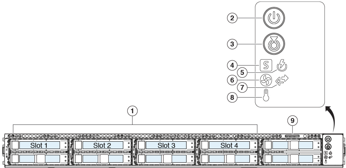
图 7: S395 前面板
