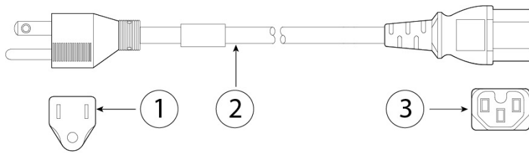
图 28: 北美 CAB-9K12A-NA
