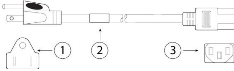
图 32: 中国台湾 CAB-ACTW
