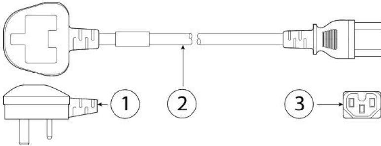
图 33: 英国 CAB-9K10A-UK
