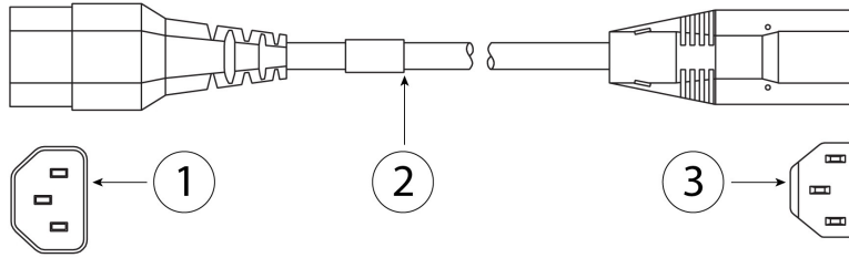
图 17: 机柜跳线 CAB-C13-C14-2M
