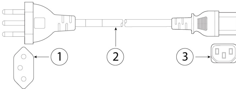
图 16: 巴西 PWR-250V-10A-BZ
