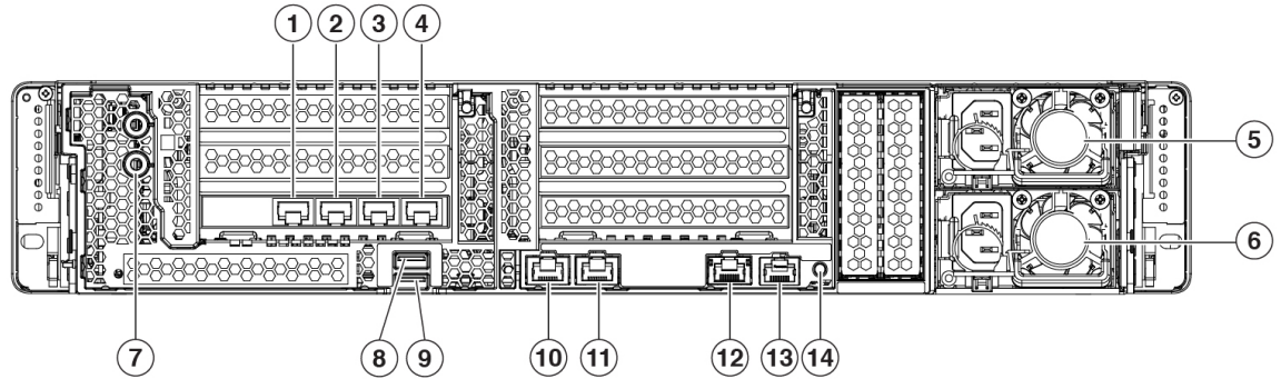
图 11: S695 后面板
