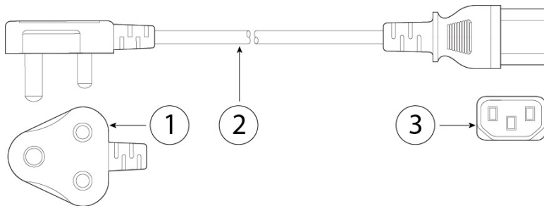
图 22: 印度 CAB-250V-10A-ID
