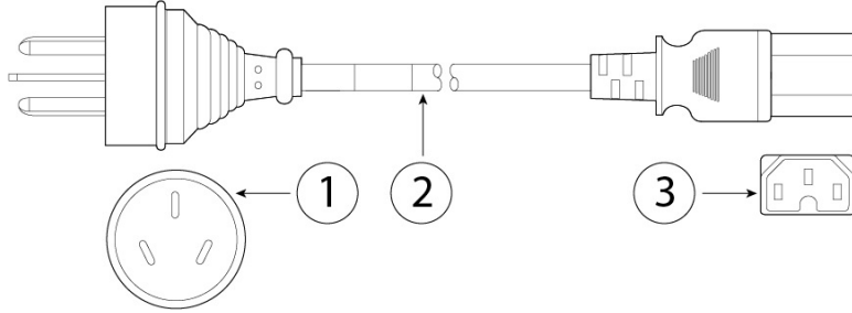
图 15: 澳大利亚 CAB-9K10A-AU
