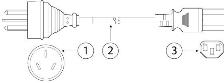
图 14: 阿根廷 CAB-250V-10A-AR
