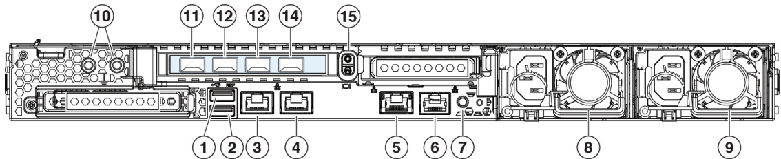
图 10: S195 和 S395 后面板
