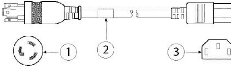
图 30: 北美 CAB-AC-L620-C13
