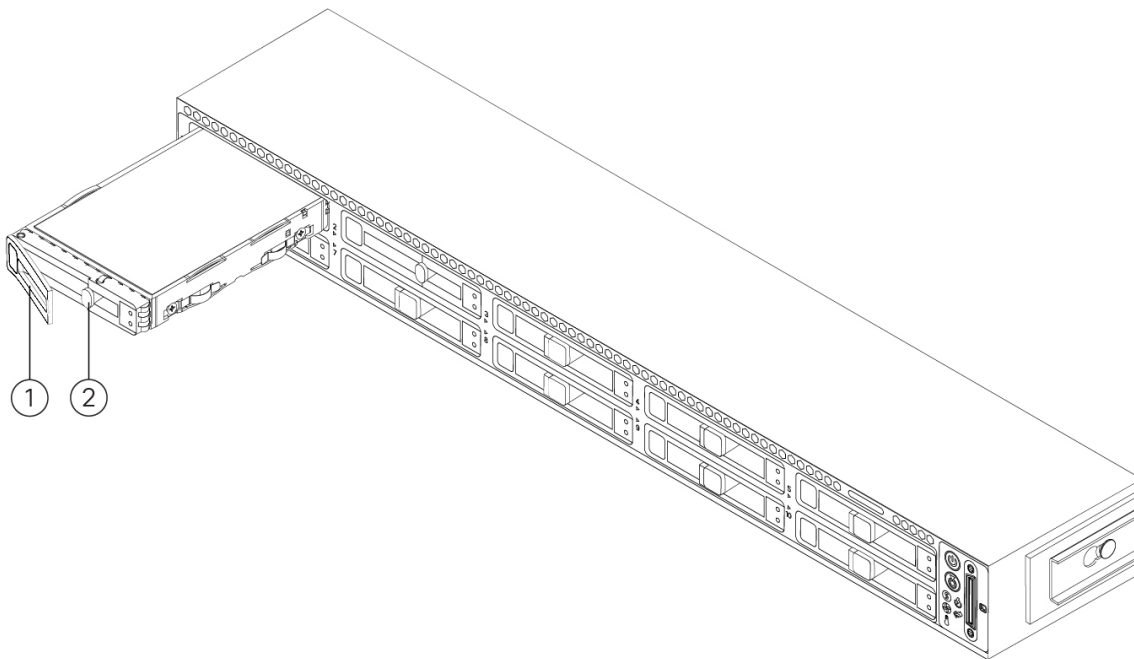
图 38: 拆卸驱动器
