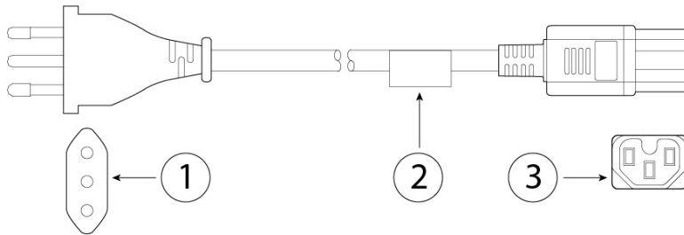
图 24: 意大利 CAB-9K10A-IT
