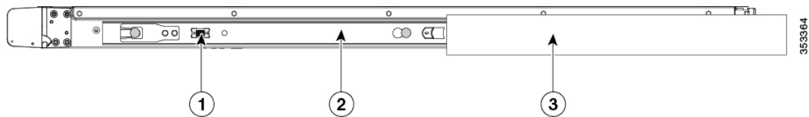
图 36: 内滑轨释放扣夹
