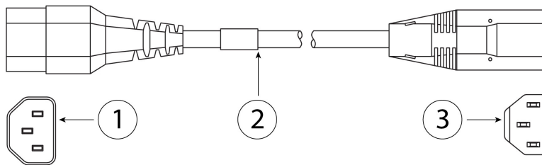
图 19: 机柜跳线 CAB-C13-CBN
