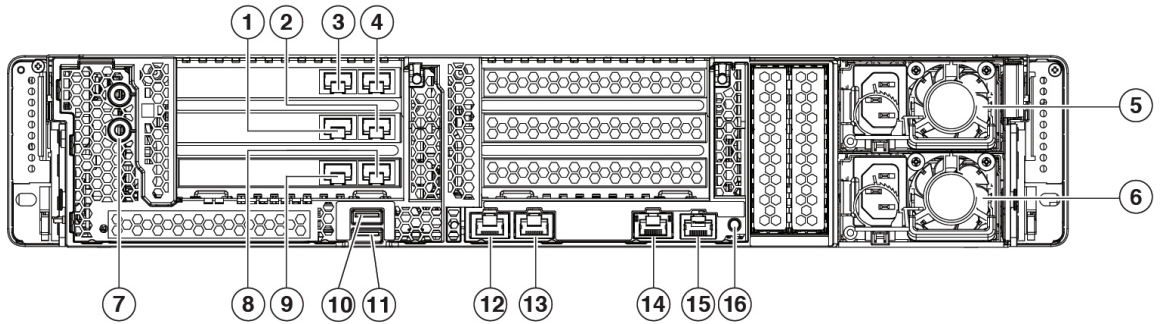
图 12: S695F 后面板
