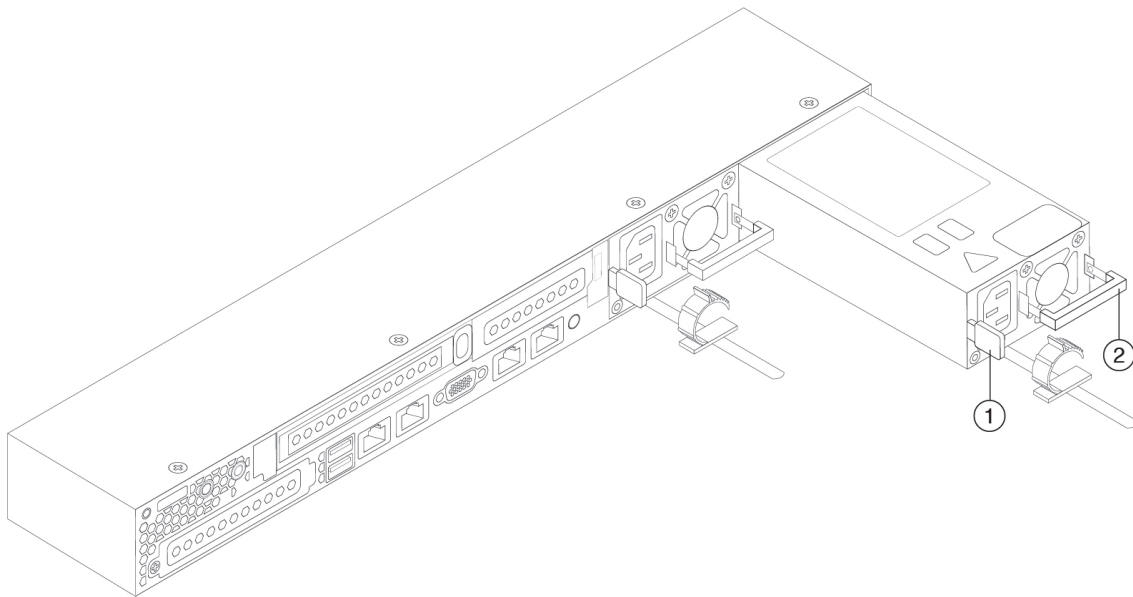
图 40: 拆卸和更换交流电源
