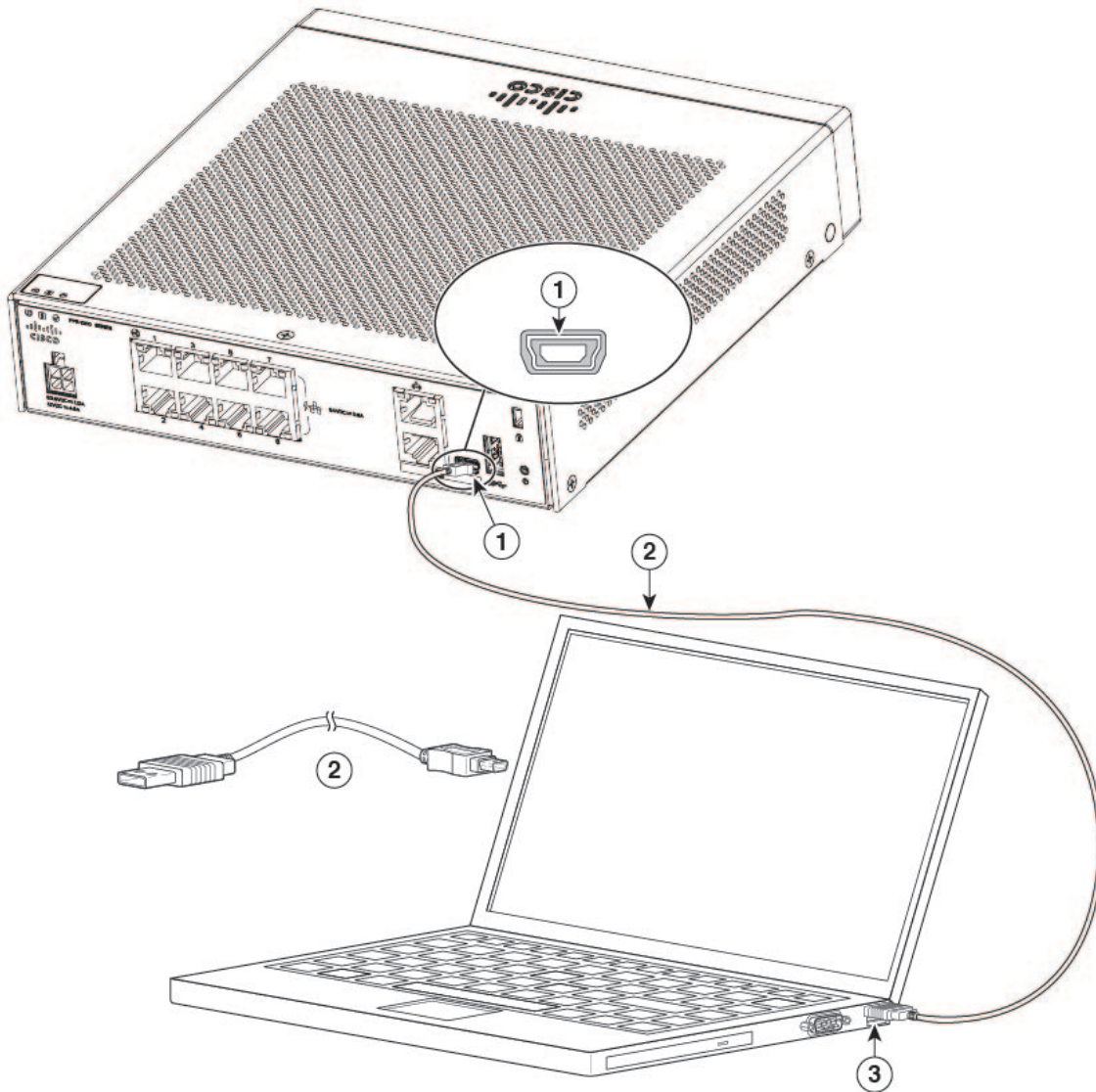
图 1: 控制台端口连接
