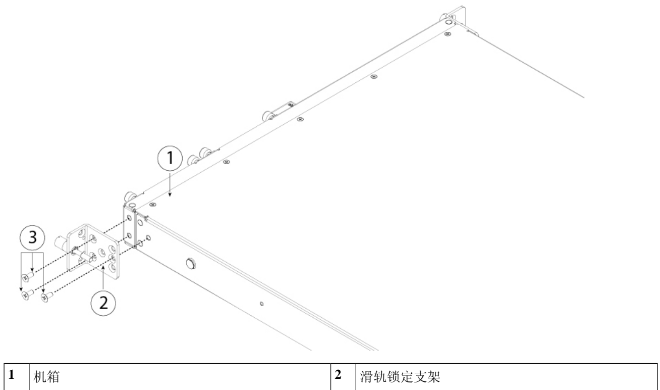
图 41: 将滑轨锁定支架固定到机箱的两侧
