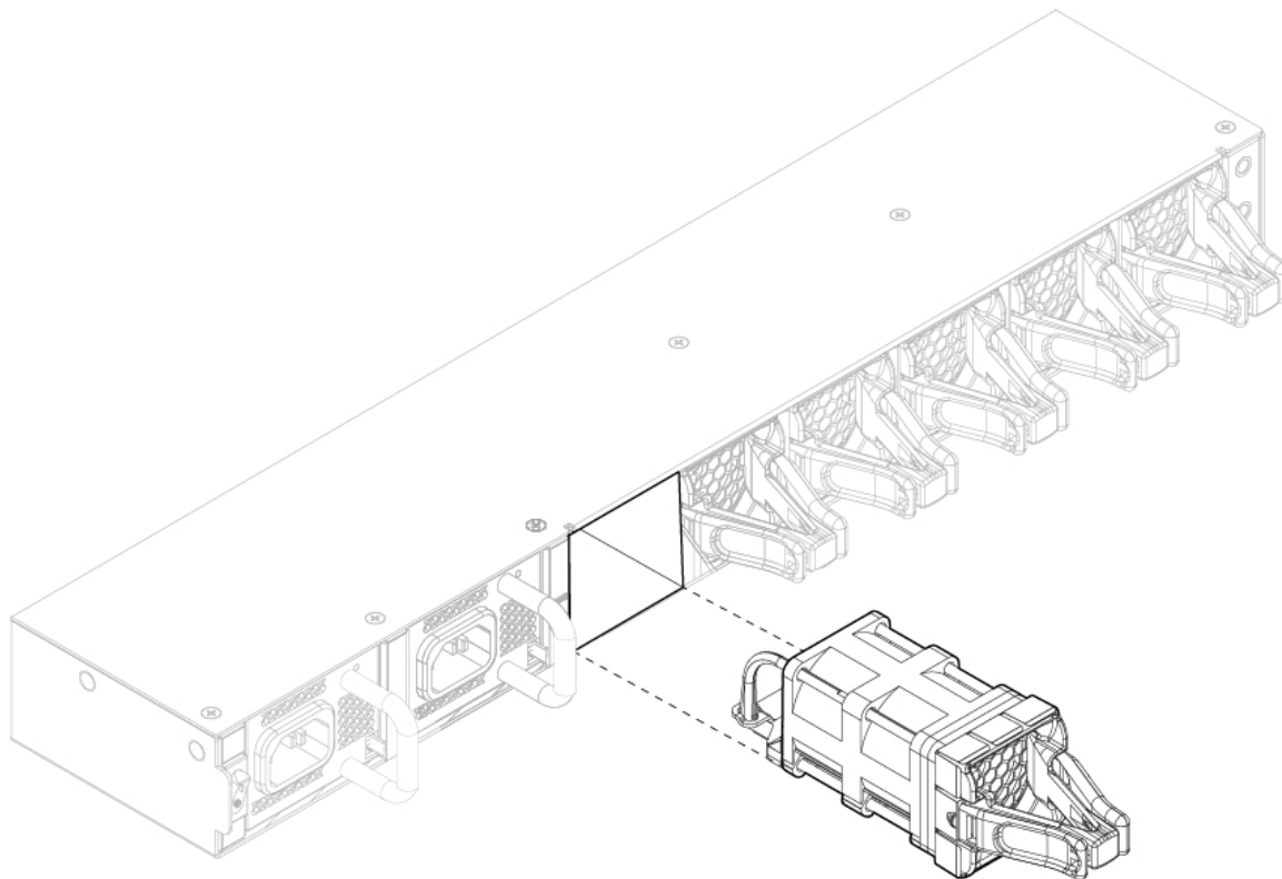
图 47: 拆卸风扇模块
