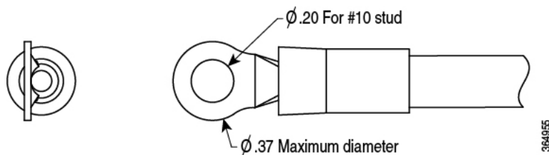
图 50: 直流电源输入电缆引线
