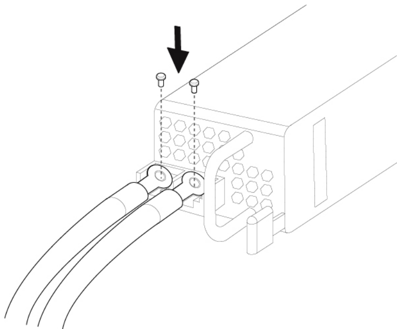
图 54: 拧紧 M5 螺钉
