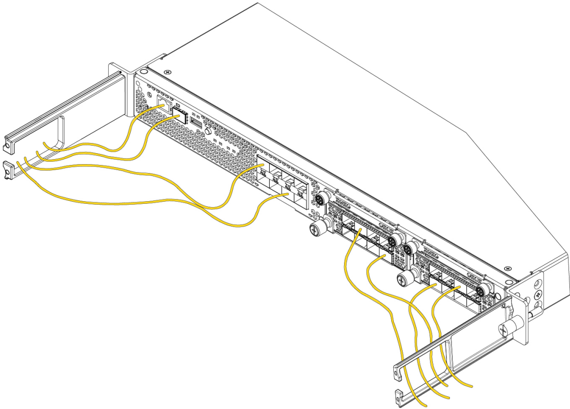
图 43: 将电缆穿过电缆管理支架
