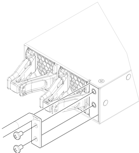
图 40: 固定接地片
