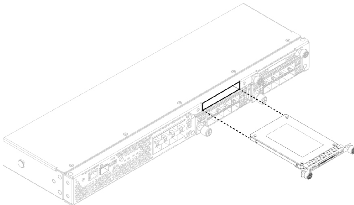
图 48: 移除 SSD
