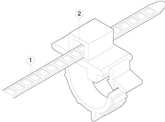
图 56: 线扣穿过线扣夹的箱形通道
