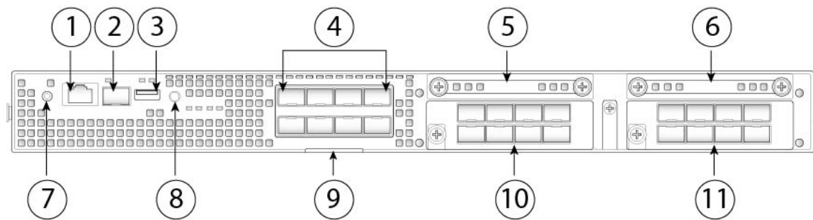
图 5: Firepower 4100 前面板
