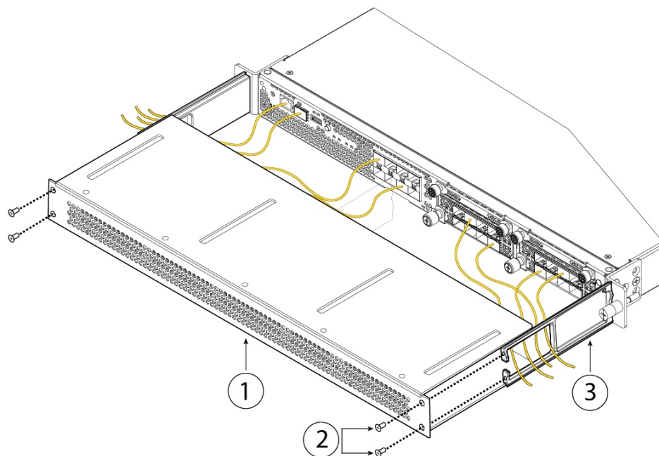
图 44: 将 FIPS 不透明防护罩固定到电缆管理支架
