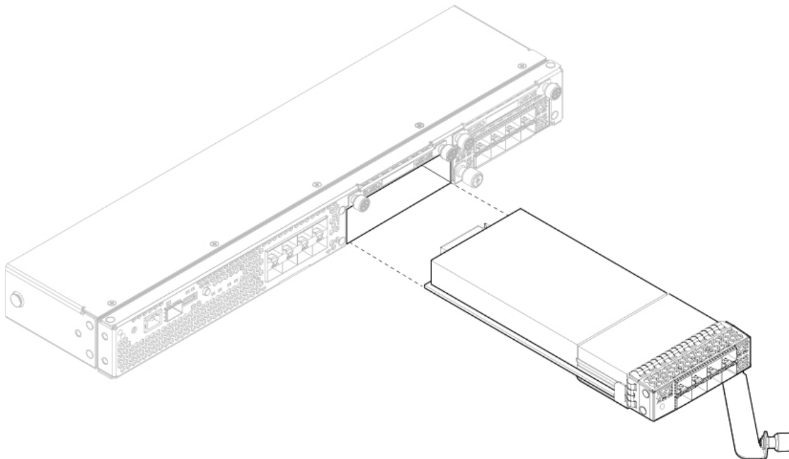
图 46: 拆卸网络模块
