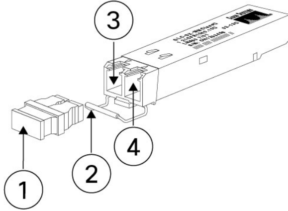
图 15: SFP
