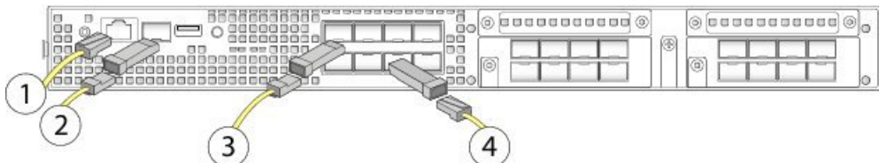
图 45: 将电缆连接到 Firepower 4100
