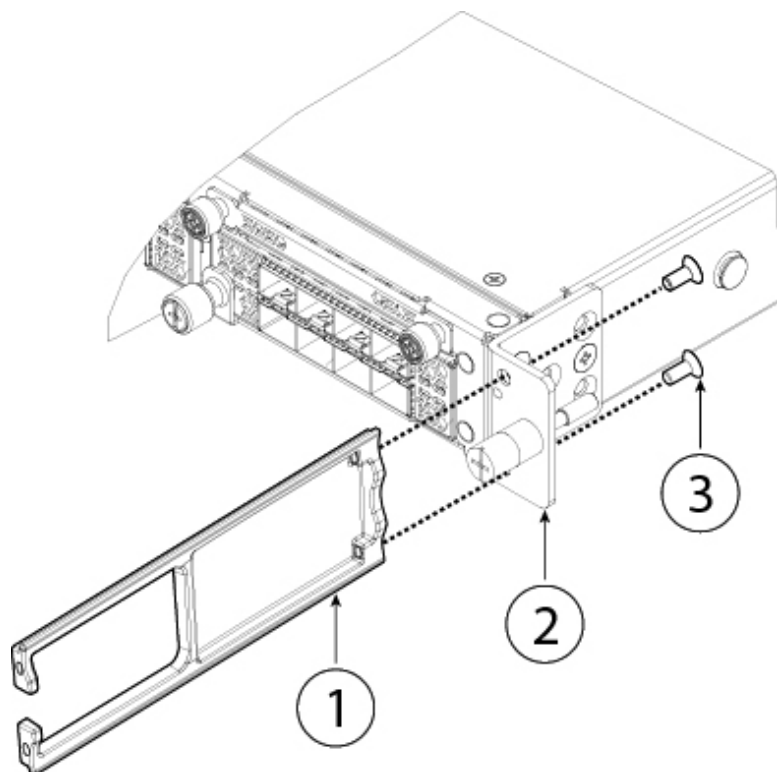
图 42: 将电缆管理托架固定到滑轨锁定支架
