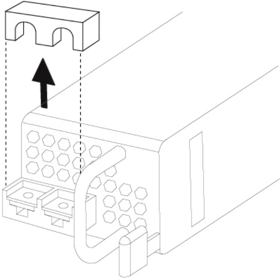
图 51: 拆卸塑料盖
