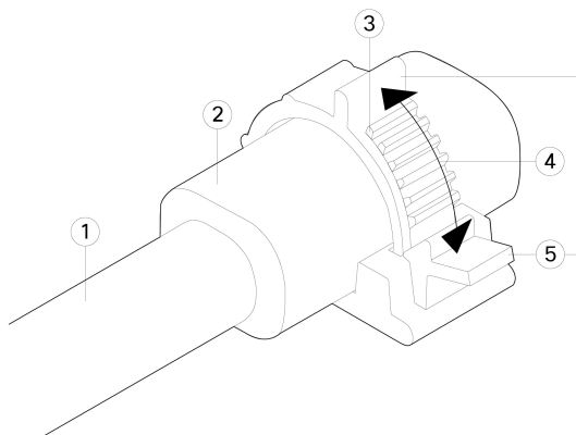
图 59: 线扣夹扣在电源线塑胶部分
