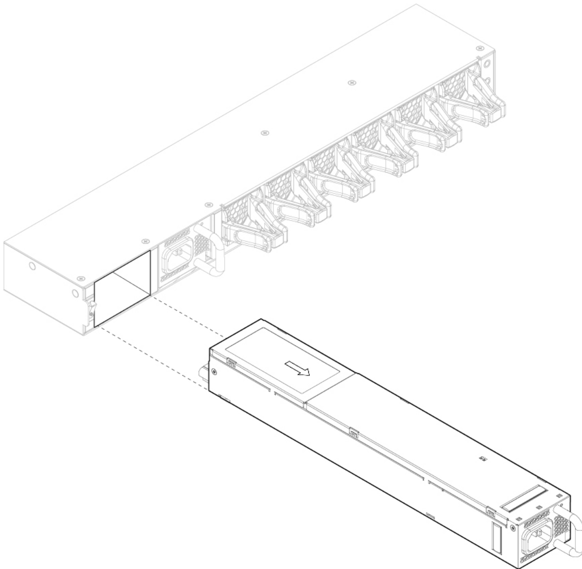
图 49: 拆卸电源模块
