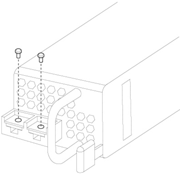
图 52: 拆卸 M5 螺钉
