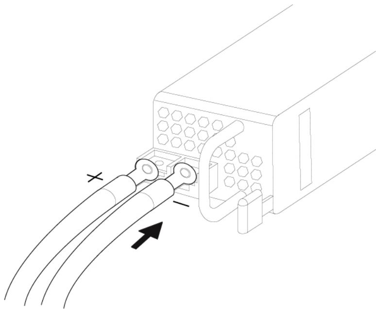
图 53: 插入电缆
