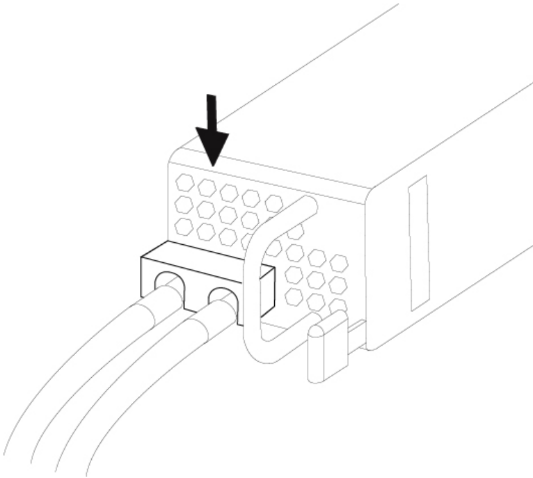
图 55: 盖上塑料盖
