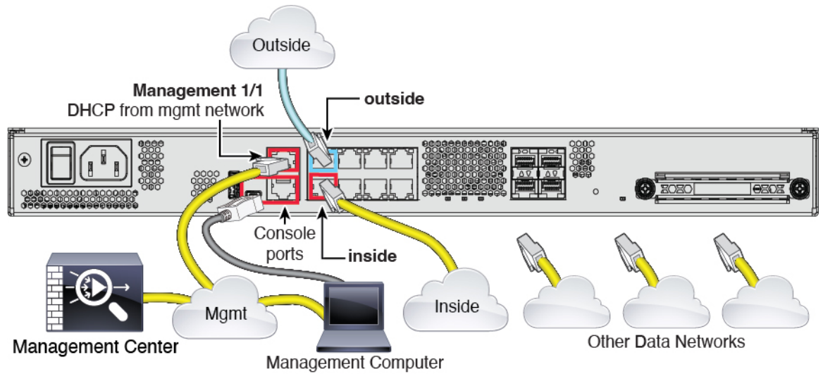
图 3: 连接单独管理网络的电缆
