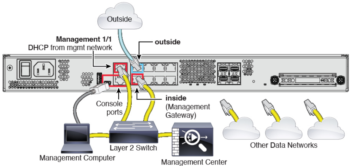
图 4: 进行边缘部署布线
