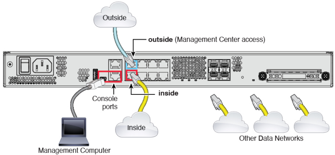
图 17: 远程管理部署的布线
