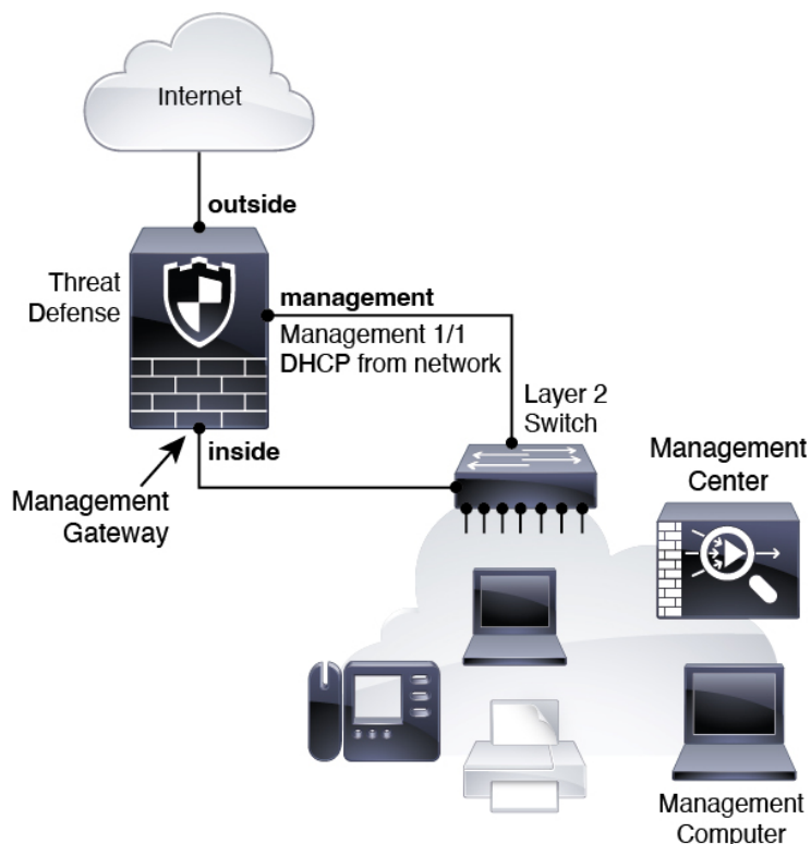
图 2: 边缘网络部署
