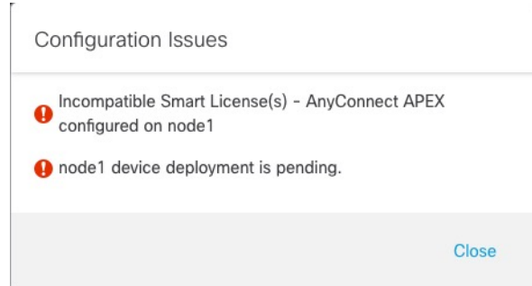
图 2: 配置问题
