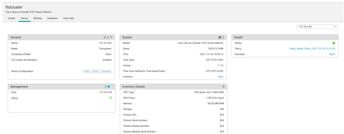
图 8: 选择节点
