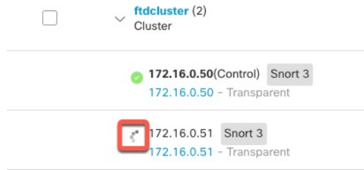
图 15: 节点注册
