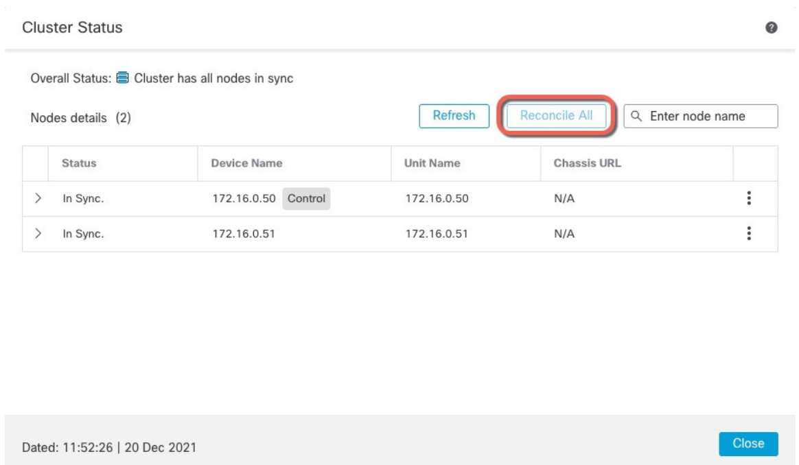
图 25: 协调全部
