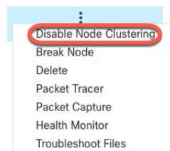
图 20: 禁用集群
