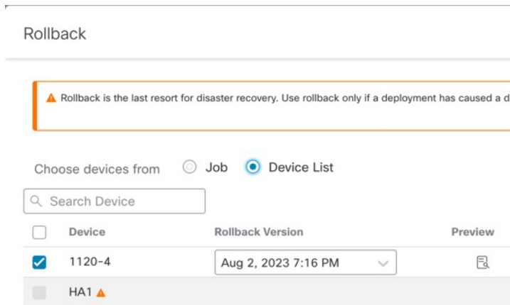
图 19: 设备列表
