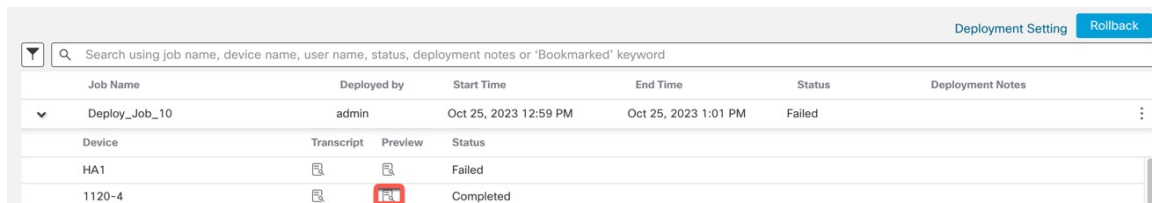
图 15: 预览图标
